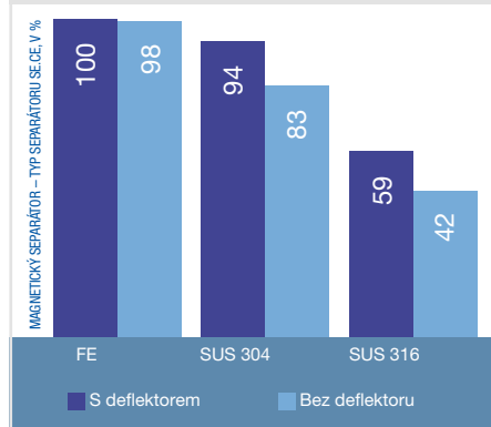
Účinnost magnetické separace pro kovové částice \varnothing 0,8 \times 2 mm
